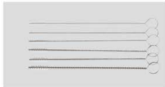
HN-120シリーズ 極細管 φ1.5～φ4.0 全長120mm
