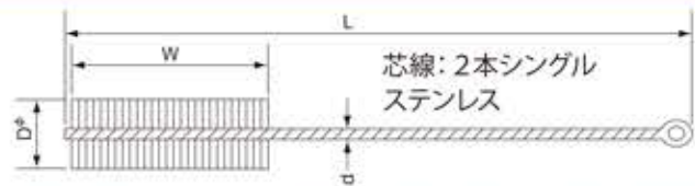
HN-120シリーズ 極細管 φ1.5～φ4.0 全長120mm
